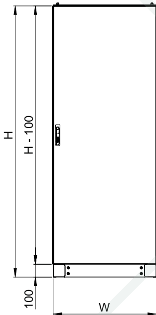
ÖN GÖRÜNÜŞ
