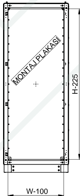
İÇ GÖRÜNÜŞ
