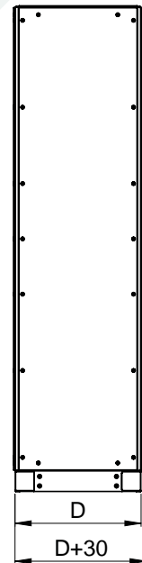
YAN GÖRÜNÜŞ
