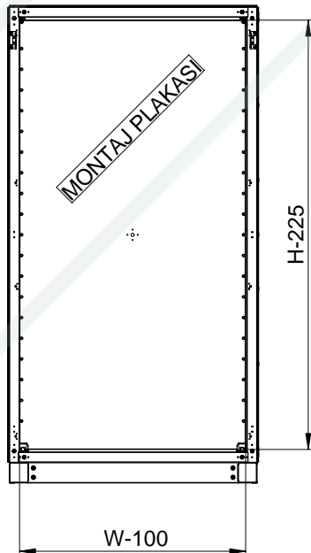
İÇ GÖRÜNÜŞ
